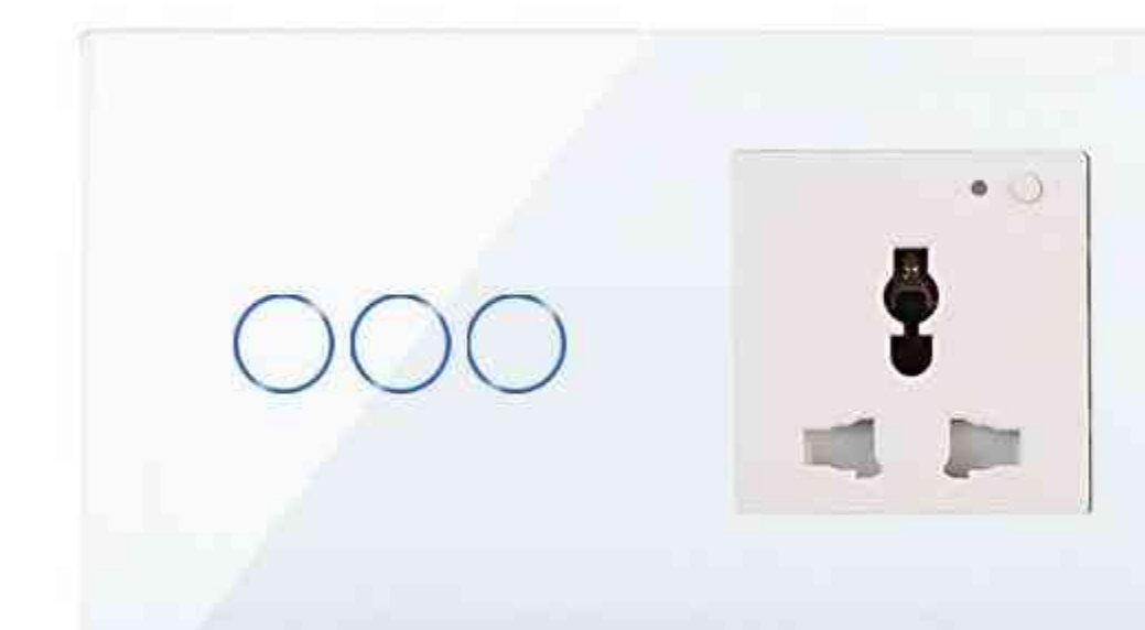
3g1w+16A universal socket 86*146 Wi-Fi/Touch/RF/ZigBee
