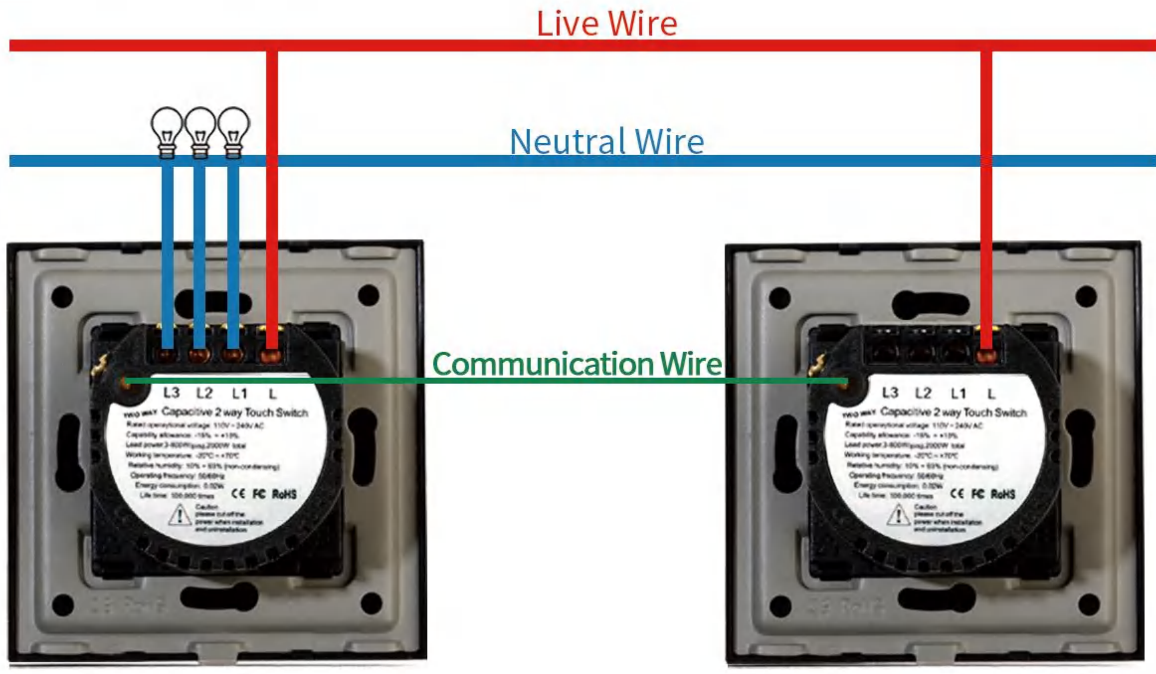
2way wiring
