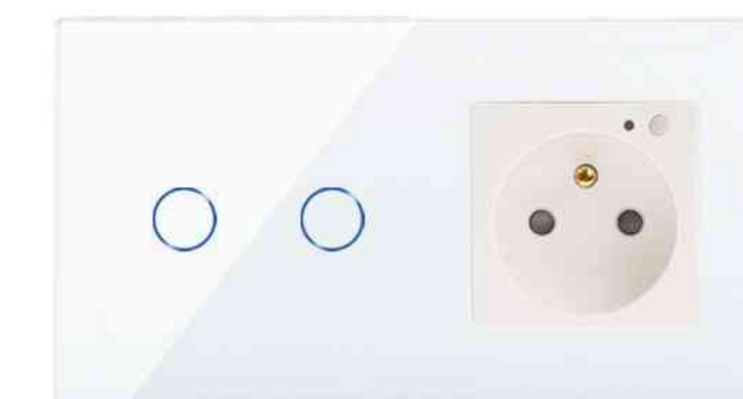
2g1w+French socket 86*157 Wi-Fi/Touch/RF/ZigBee
